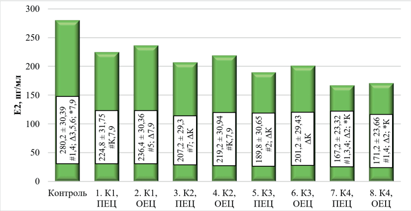
Рис. 2. Динаміка змін рівнів естрадіолу при застосуванні циклофосфаміду в експерименті: K1–K4 – курси введення препарату; ПЕЦ – перший естральний цикл після відповідного курсу; ОЕЦ – останній естральний цикл після відповідного курсу та перед наступним курсом. Статистично достовірні різниця стосовно зазначених груп із відповідним номером: # – p<0,05 ; Δ – p<0,01 ; * – p<0,001
