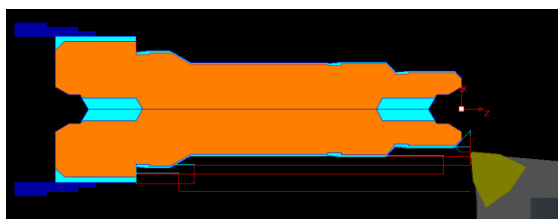
Рис. 5. Траєкторія руху інструменту при чорновій обробці поверхонь
