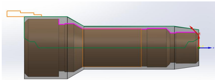
Рис. 1. Імпортована деталь та заготовка з контуром поверхні деталі, який потрібно отримати після обробки
