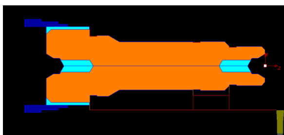
Рис. 7. Траєкторія руху інструменту при нарізанні канавок
